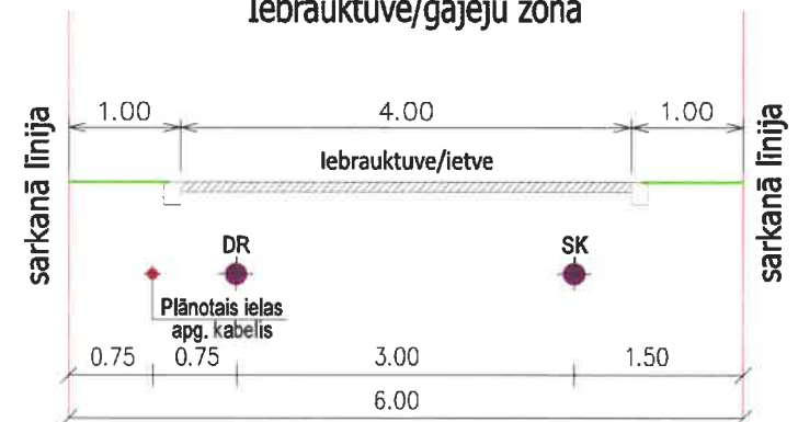
GRIEZUMS 3 - 3 M1:50 Iebrauktuve/gājēju zona
