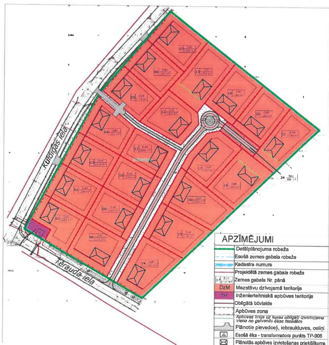
22. att. Detālplānojuma teritorijas apbūves struktūras priekšlikums
