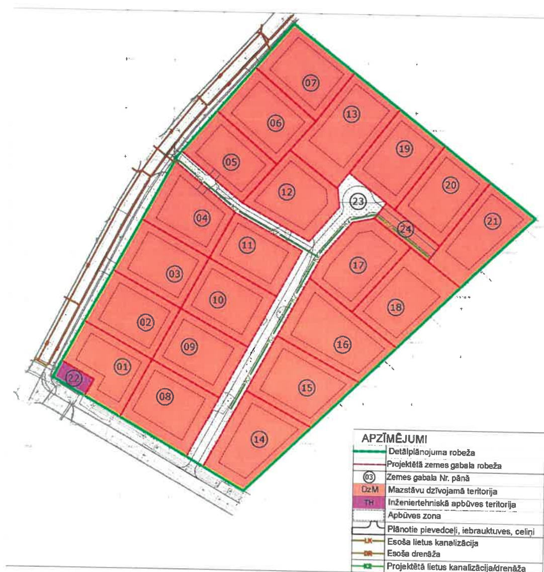
26. att. Deālplānojuma teritorijas ūdensatvades risinājums
