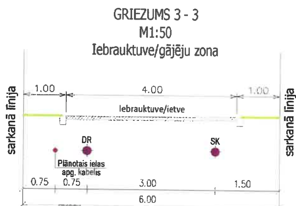
29. att. Plānoto komunikāciju izvietojums pievedceļa, pievedceļa un gājēju celiņa/ietves teritorijā (šķēršprofils)
